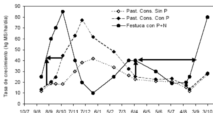
Figura 2: Distribución estacional del crecimiento de una pastura asociada con y sin aplicación de P y de una pastura de festuca con aplicación de P y de N. Las flechas destacan los efectos de la fertilización (ver texto).
